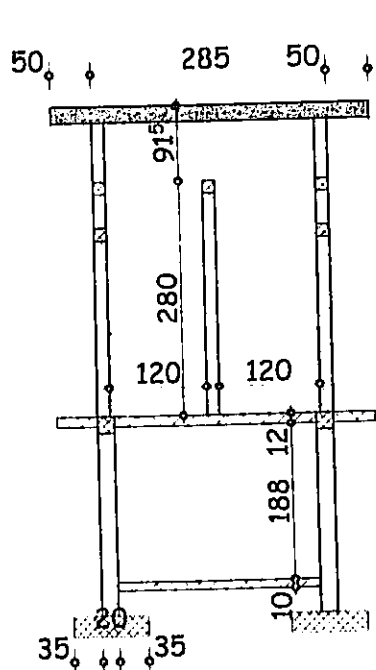
COUPE B-B
