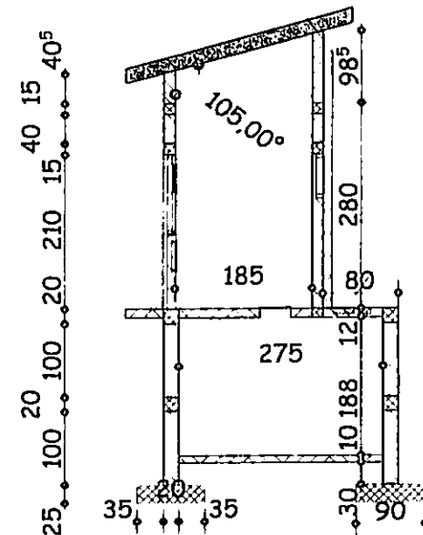
COUPE A-A
