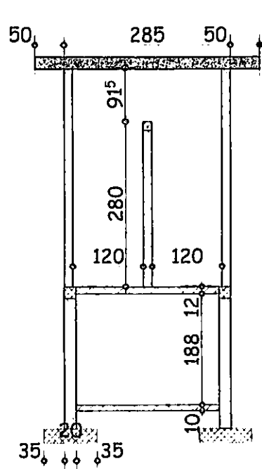
COUPE B-B
